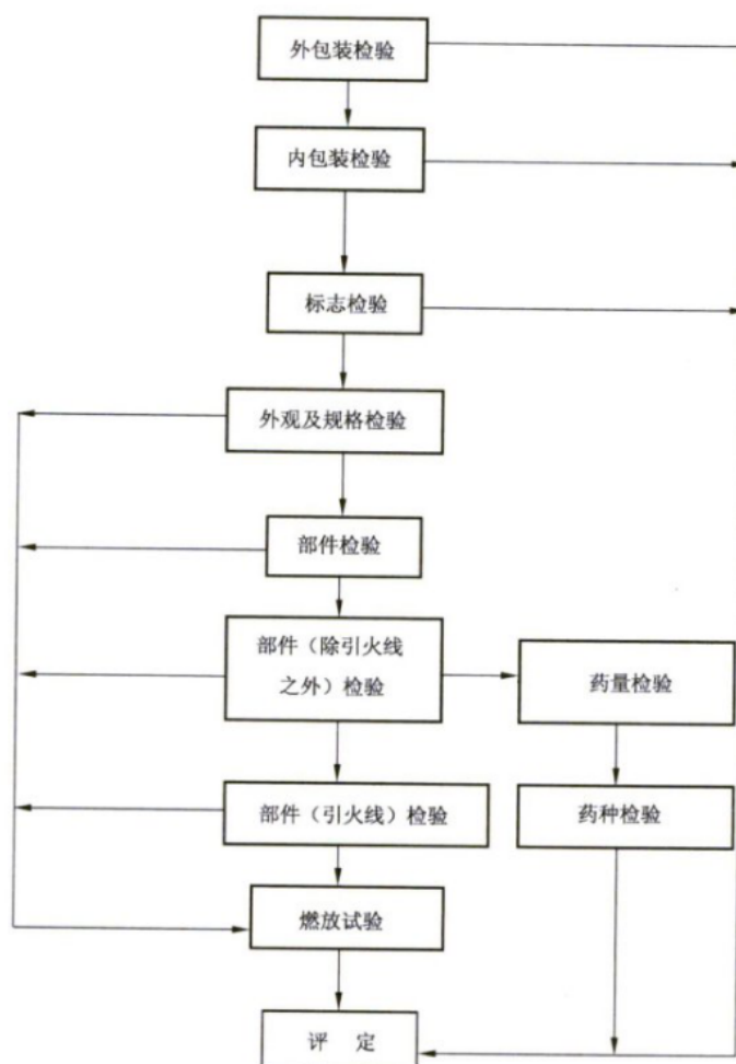
图 1 大型地面礼花检验评定流程
